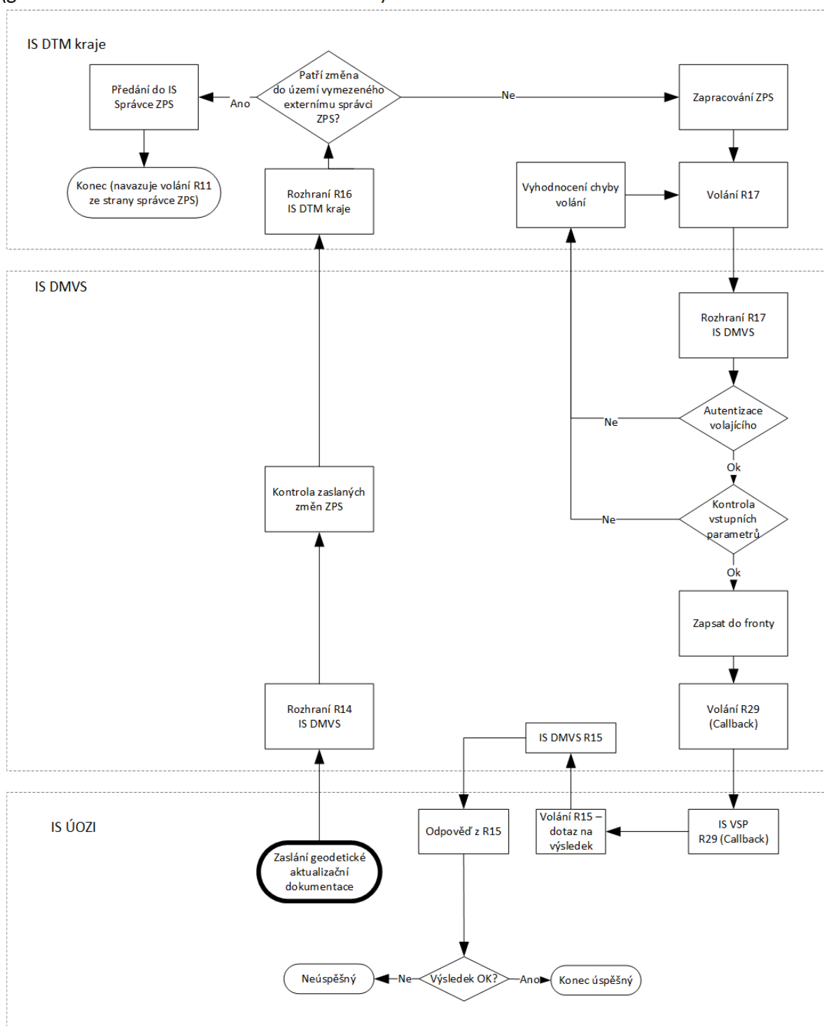
obr: Schéma workflow příjmu aktualizací geodetických podkladů
