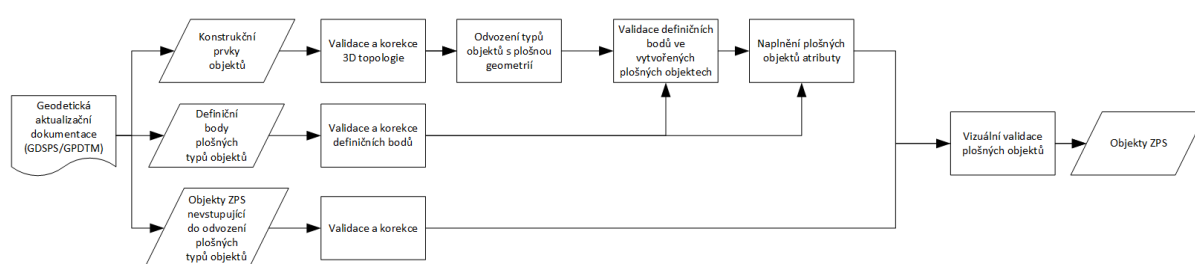
Obr. Schéma postupu odvozování plošných typů objektů
