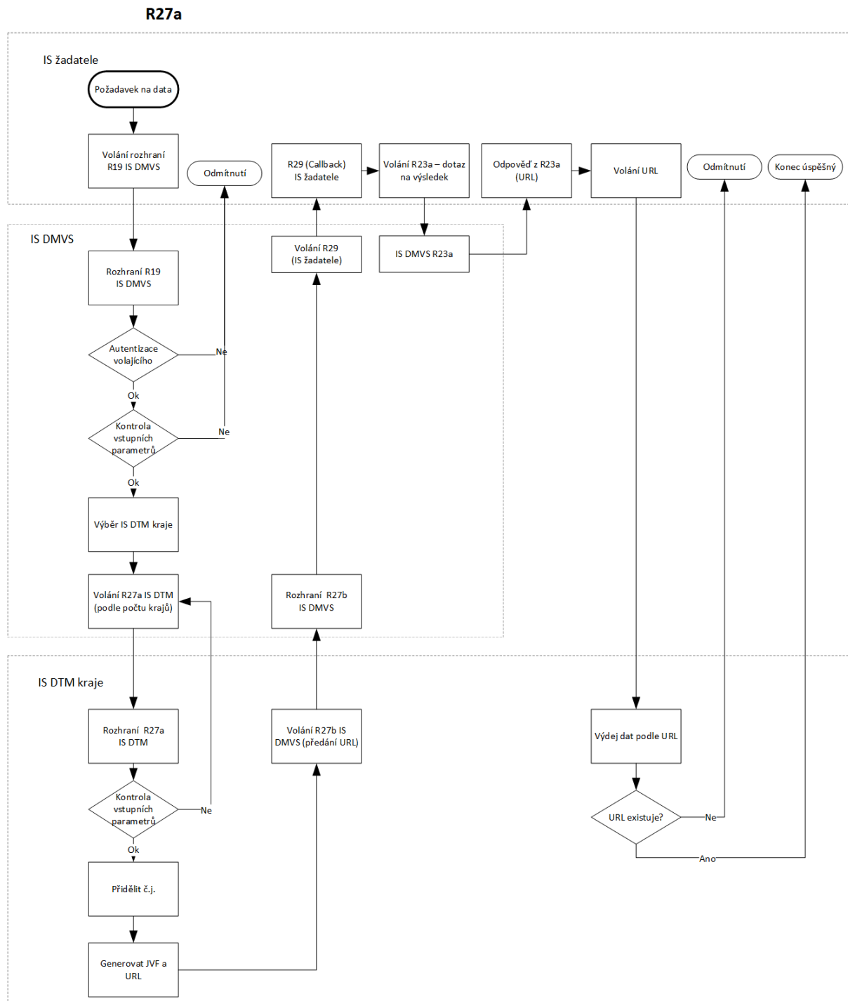
obr. schéma workflow služby R27 k poskytování dat - Služba pro vyhotovení JVF dle zadaných parametrů
