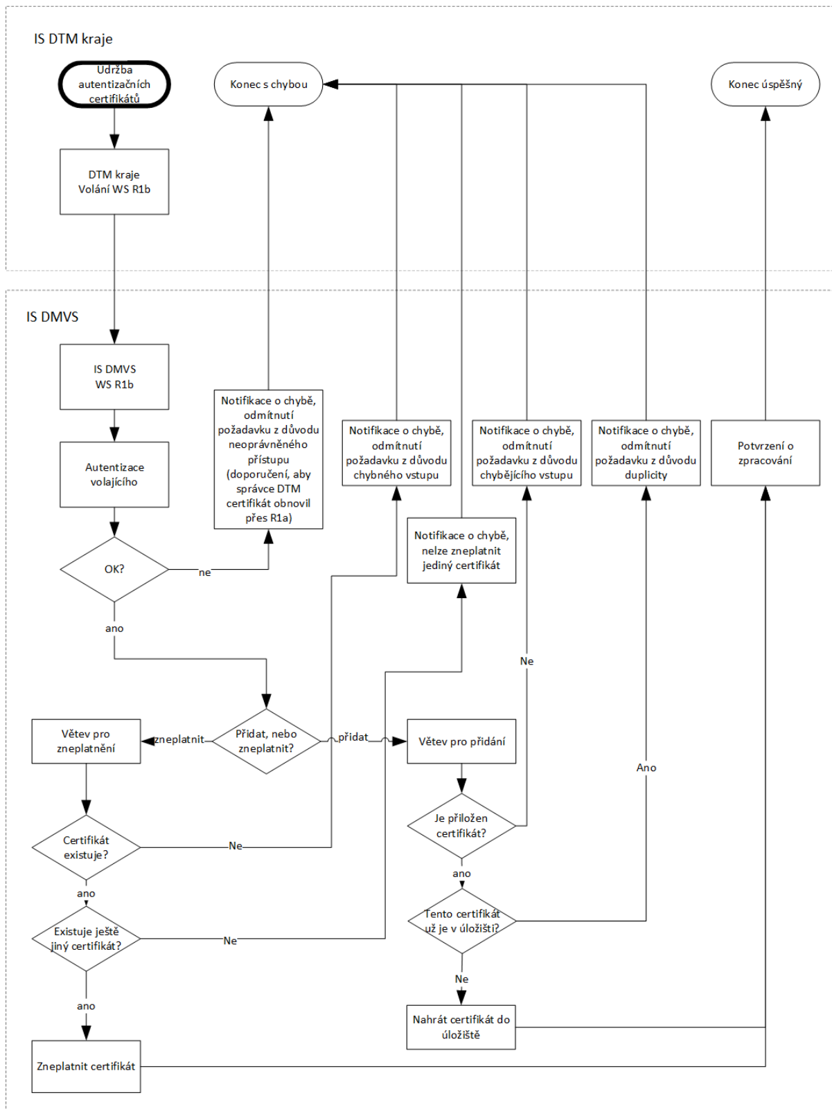
obr: Schéma registrací (certifikátů) pro využívání webových služeb
