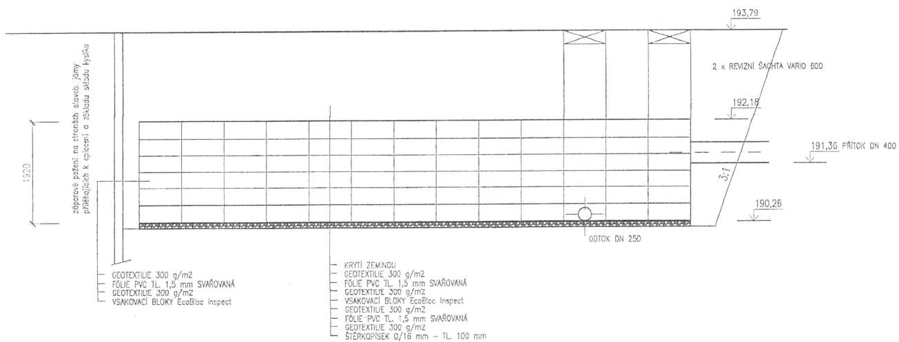
ŘEZ A-A M1:50
