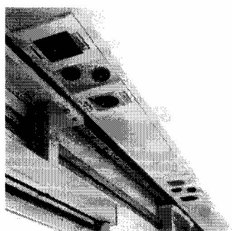
pohled na pojezd polic a připojení ze spodu mostu
