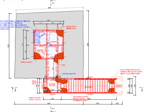
Půdorys nástupní podesty (úroveň +4170 m) (nosná k-ce)
