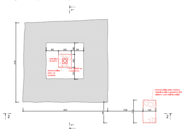
Půdorys základů (úroveň: ±0,000)
