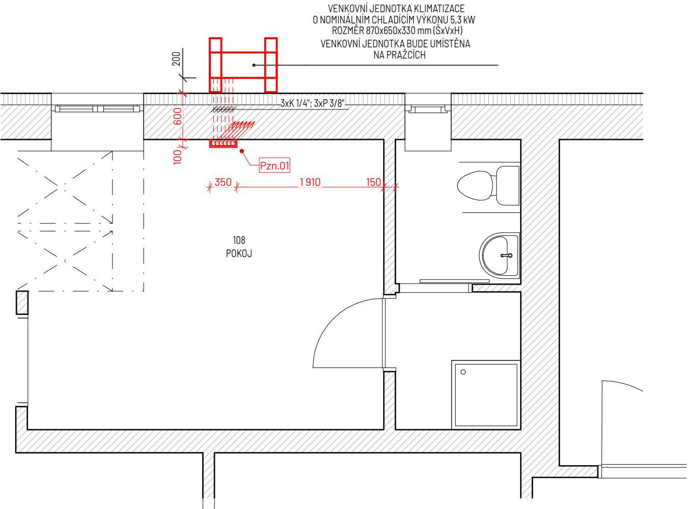
detail napojení venkovní jednotky, m=1:50
