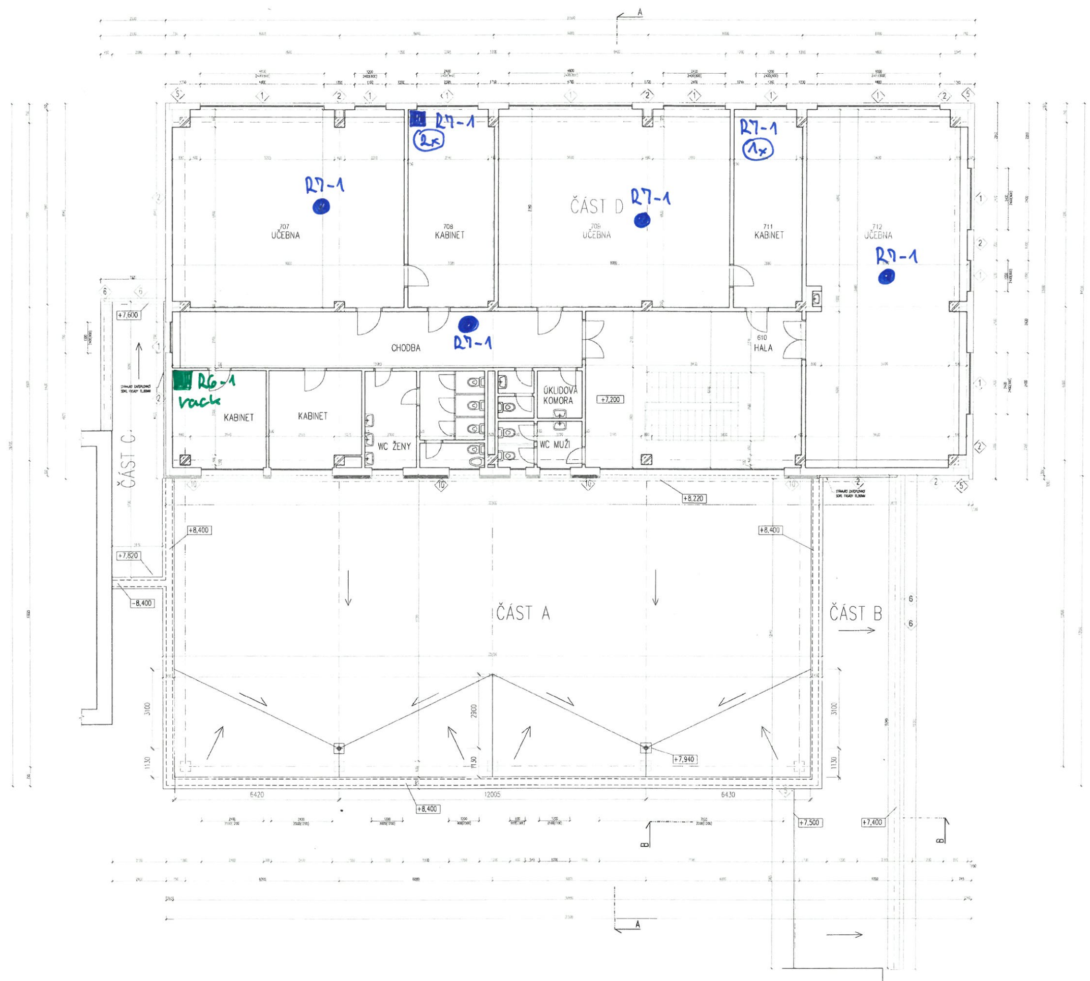
PŮDORYS 3.NP-PRĚSTAVBA
