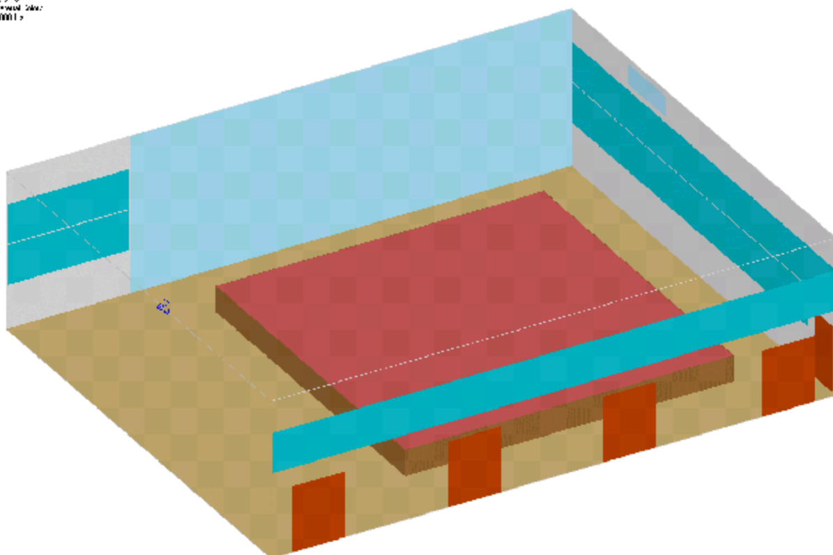
Obr. 4: Příklad vhodného umístění stěnových panelů v multifunkčním sále (m. č. 3.10).
