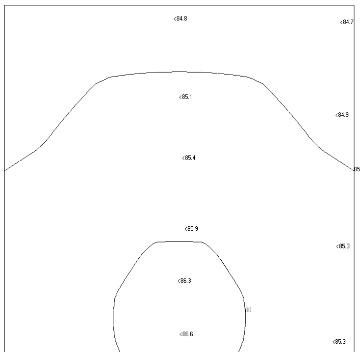
Obr. 9: Rozložení akust. hladin v poslechové ploše, multifunkční sál, zdroj – repro Dynacord CPS 320.
