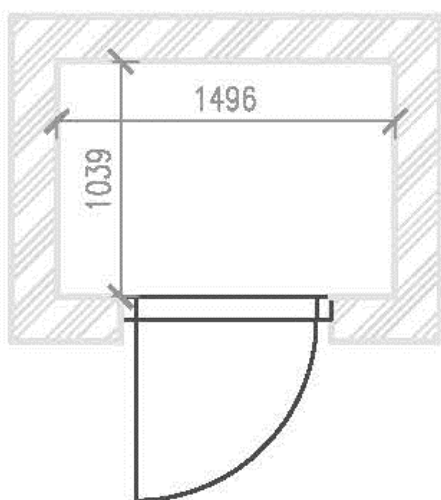
Osobní výtah OV1
