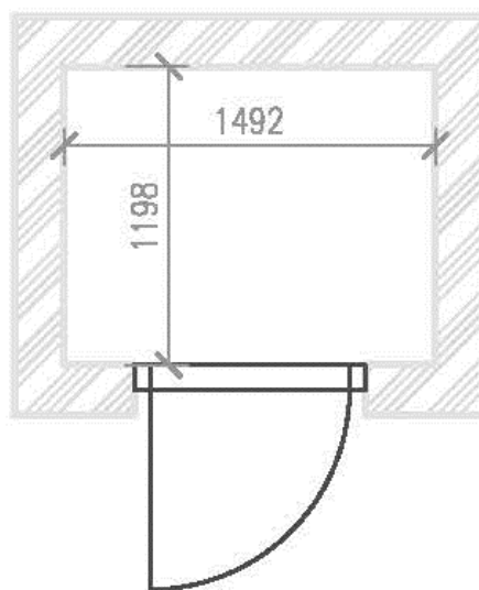
Osobní výtah OV2
