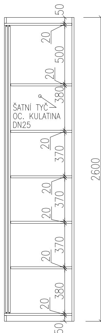
ŘEZ A
