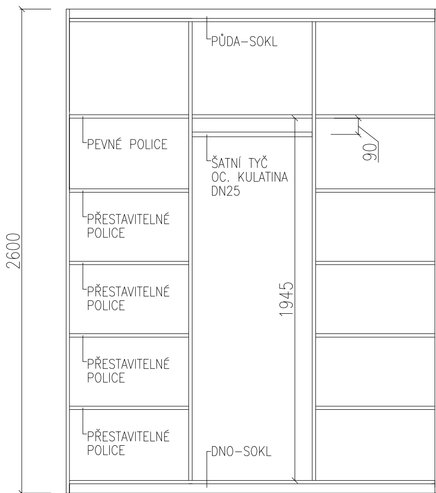
POHLED NA VESTAVĚNOU SKŘÍŇ
