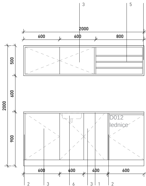
F001-KUCHYŇSKÁ LINKA-SANITKY
