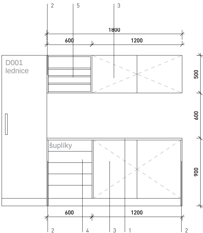
F004-LINKA LÉKÁRNA
