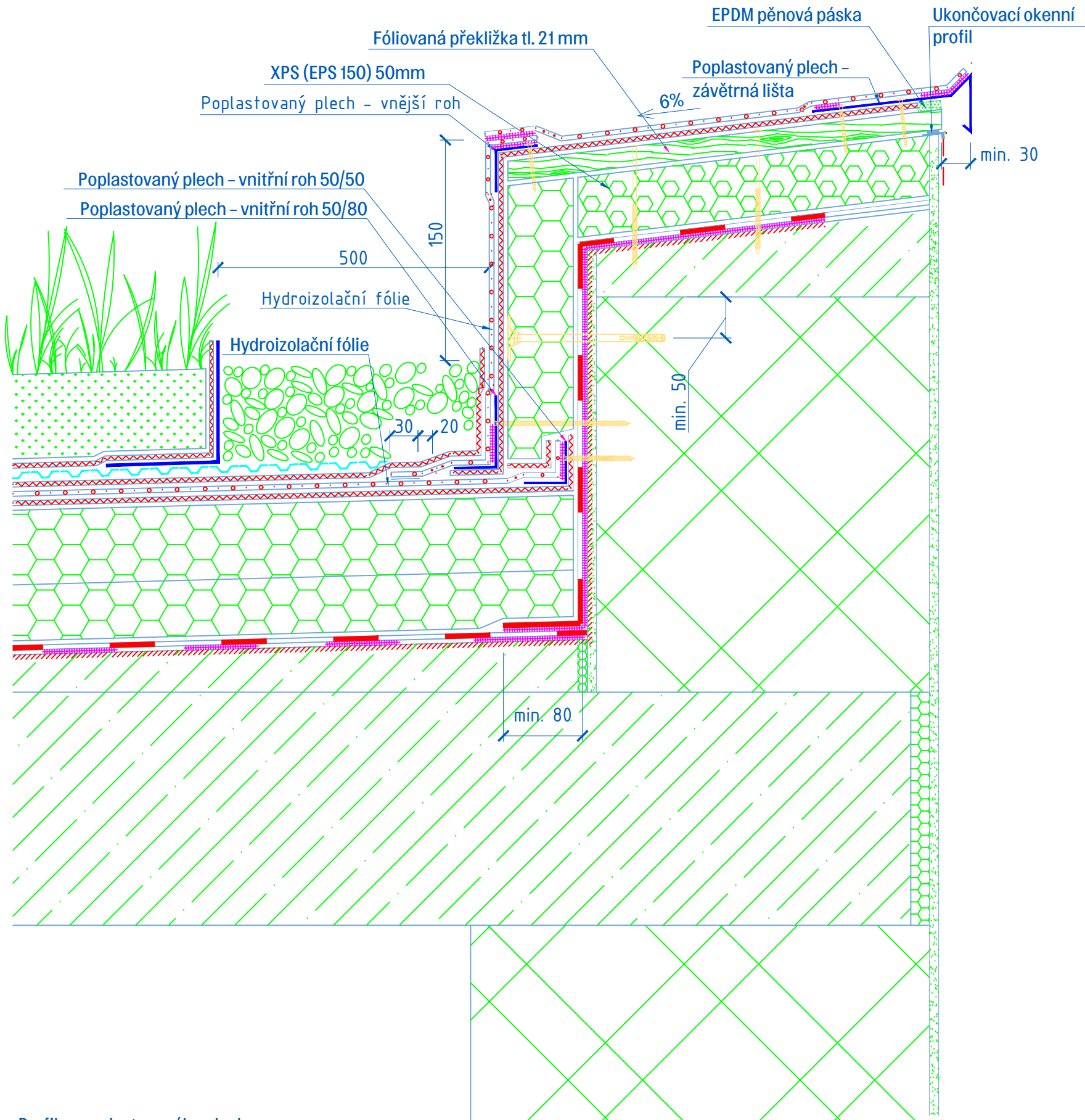
Profily z poplastovaného plechu
