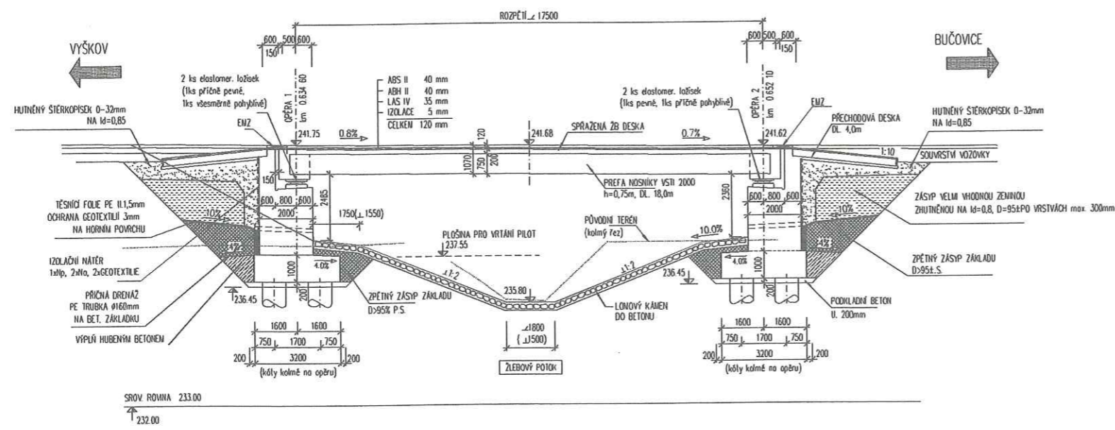
PODÉLNÝ ŘEZ MOSTEM NA SILNICI II/431, M 1:200
