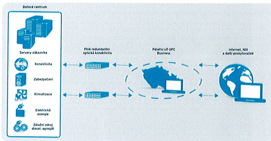
Obr. 1: Základní topologie služby UPC Business Housing
