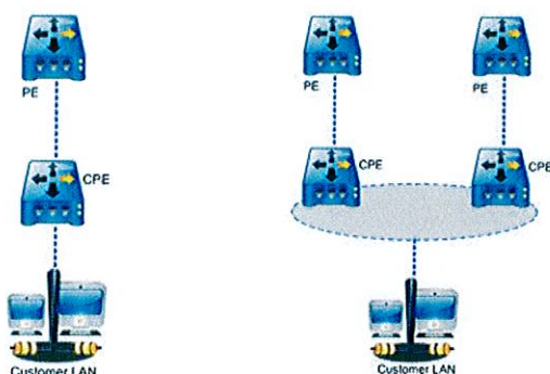
Obr1.: Dostupnost - Single Access
