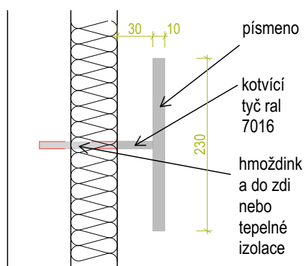
detail - řez ukotvení písmena
