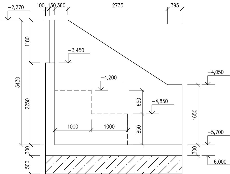
ŘEZ 2 /1:50/
