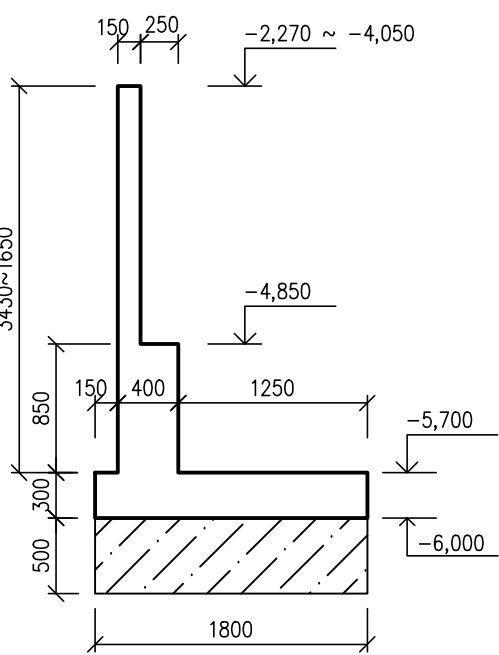
ŘEZ 4 /1:50/
