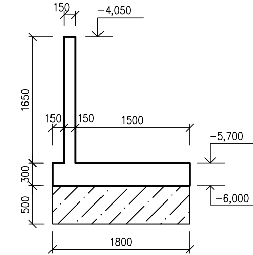
ŘEZ 5 /1:50/
