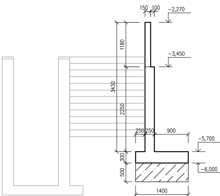
ŘEZ 2 /1:50/
