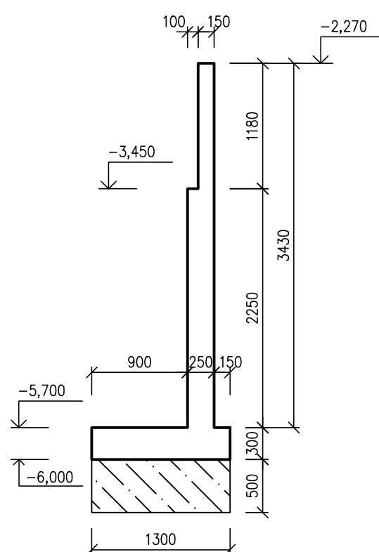
ŘEZ 3 /1:50/
