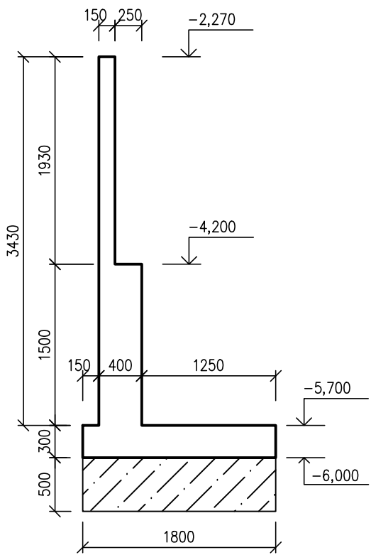
ŘEZ 3 /1:50/
