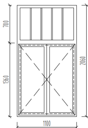
POHLED Z INTERIÉRU
